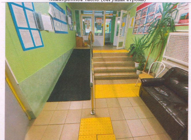
Фото № 15 – Пути движения внутри здания (лестницы). Контрастная противоскользящая лента. Указатели начало/окончания поручней. Пандус.
