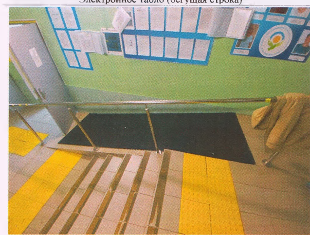
Фото № 16 – Пути движения внутри здания (лестницы). Тактильные напольные указатели. Пандус.
