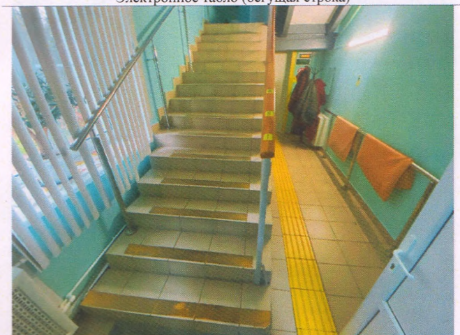
Фото № 15 – Пути движения внутри здания (лестницы). Контрастная противоскользящая лента. Указатели начало/окончания поручней.
